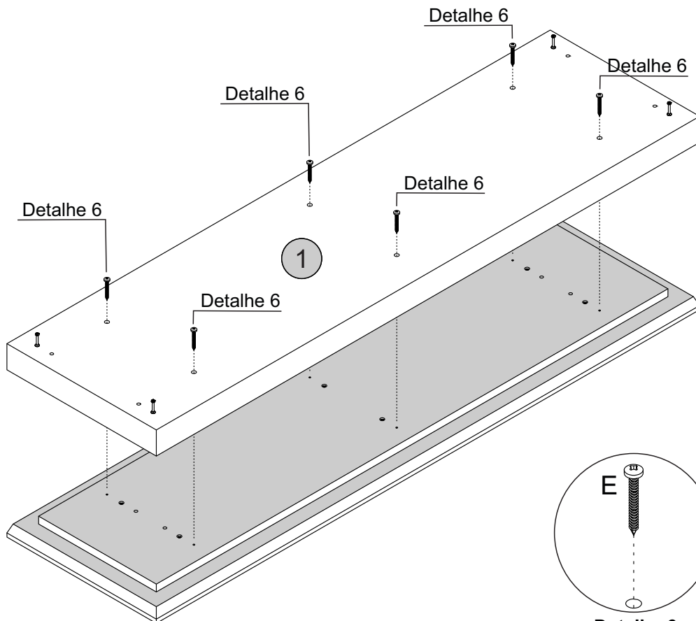
Detalhe 6 Detail/Detalle
