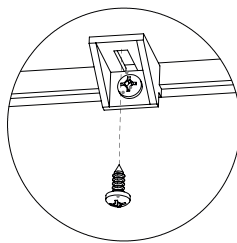
Detalhe 19 Detail/Detalle
