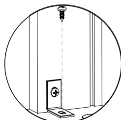
Detalhe 18 Detail/Detalle
