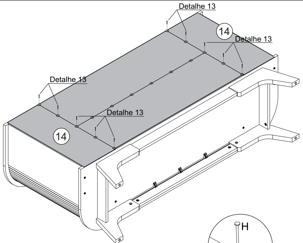
Detalhe 13 Detail/Detalle
