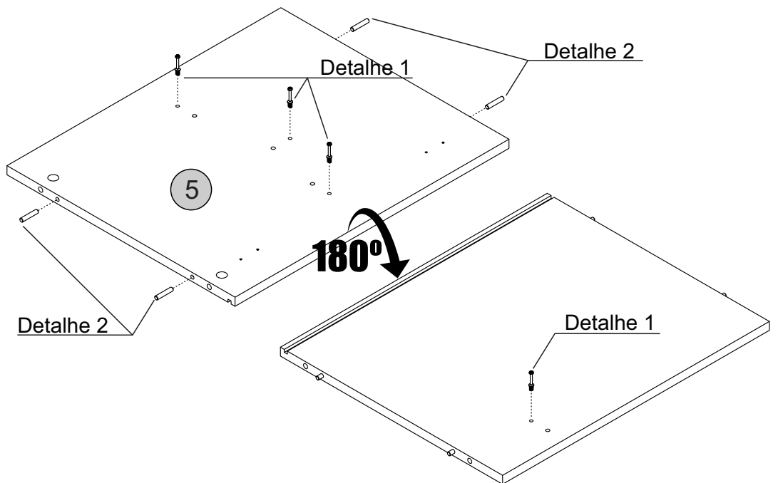
Detalhe 2 Detail/Detalle
