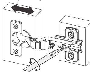
Porta Puerta Door Ajuste de profundidade Ajuste de profundidad Depth adjustment
