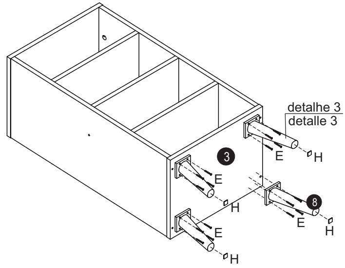
detalhe/detalle 3
