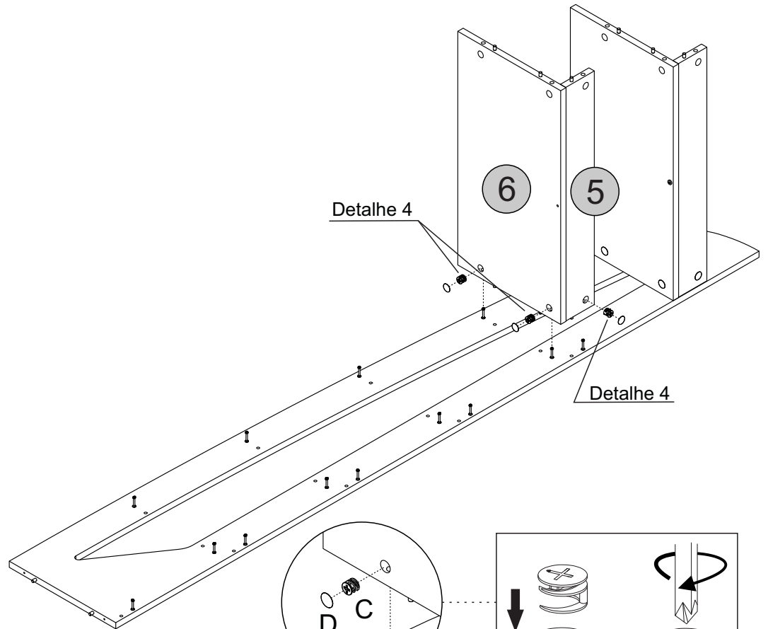
Detalhe 4 Detail/Detalle
