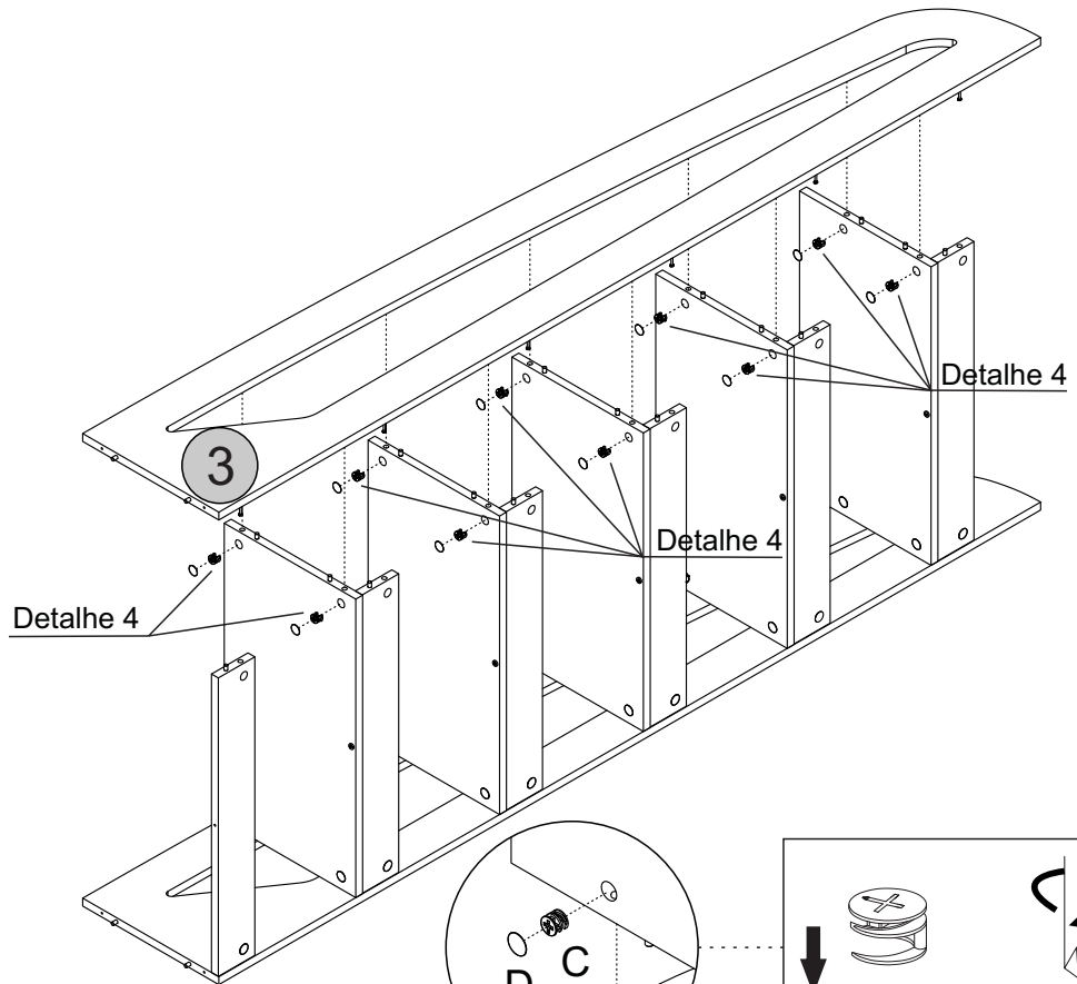
Detalhe 4 Detail/Detalle
