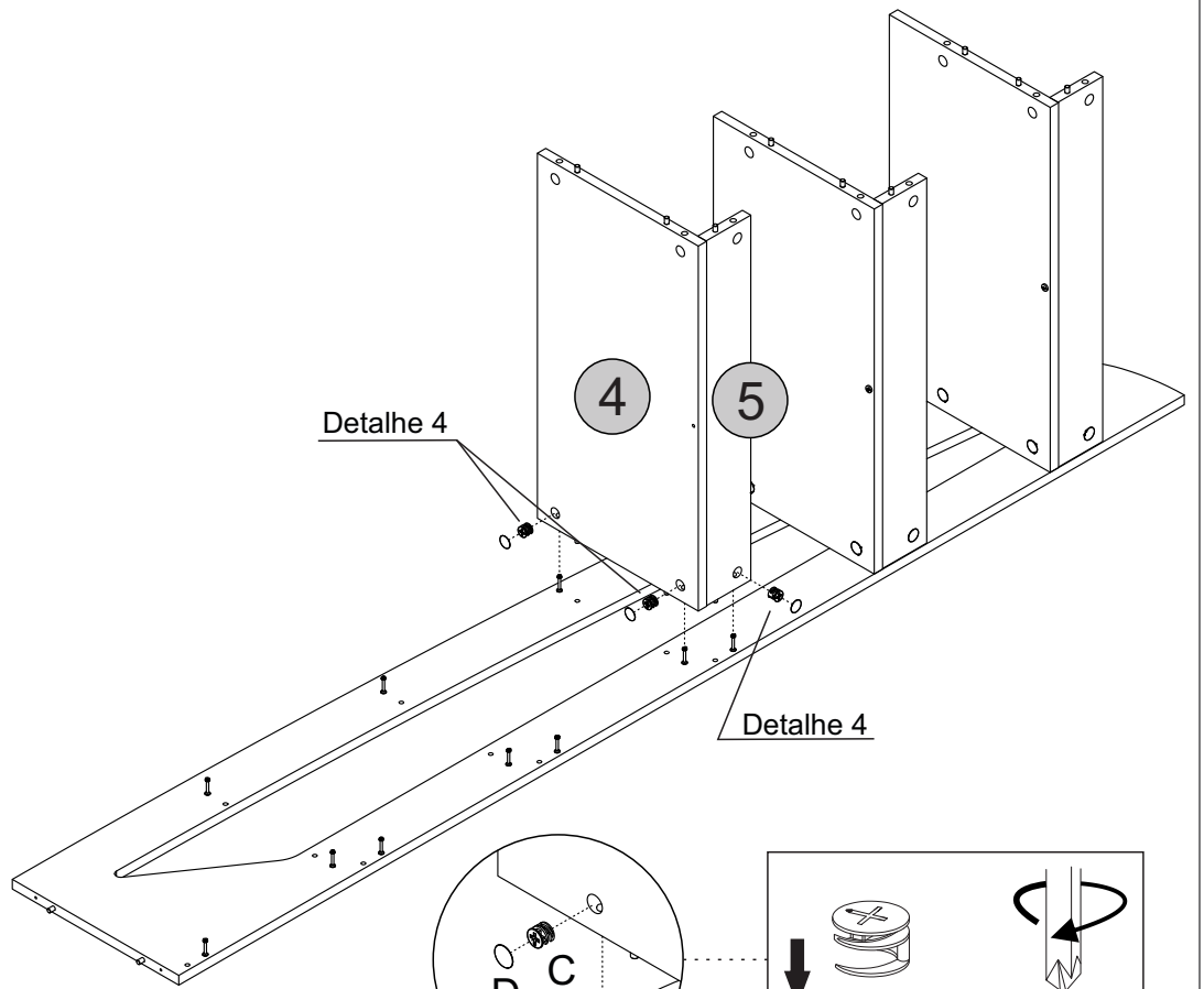
Detalhe 4 Detail/Detalle
