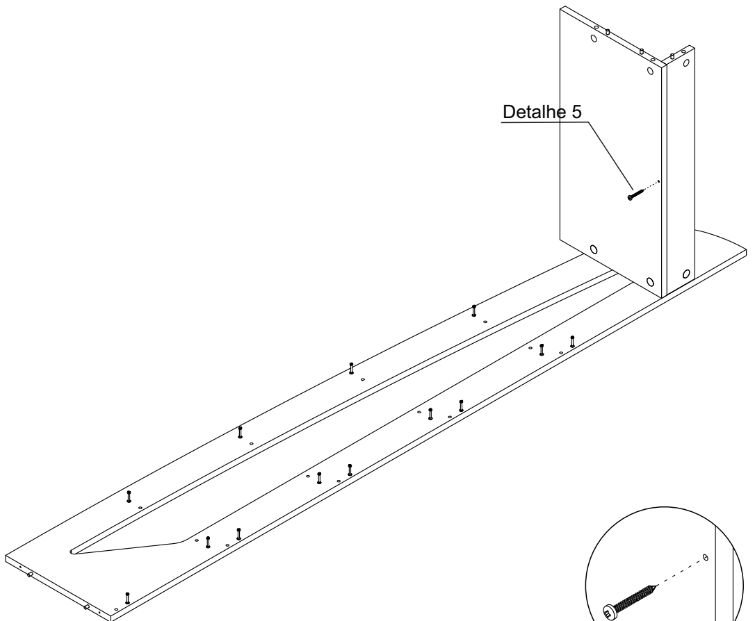
Detalhe 5 Detail/Detalle
