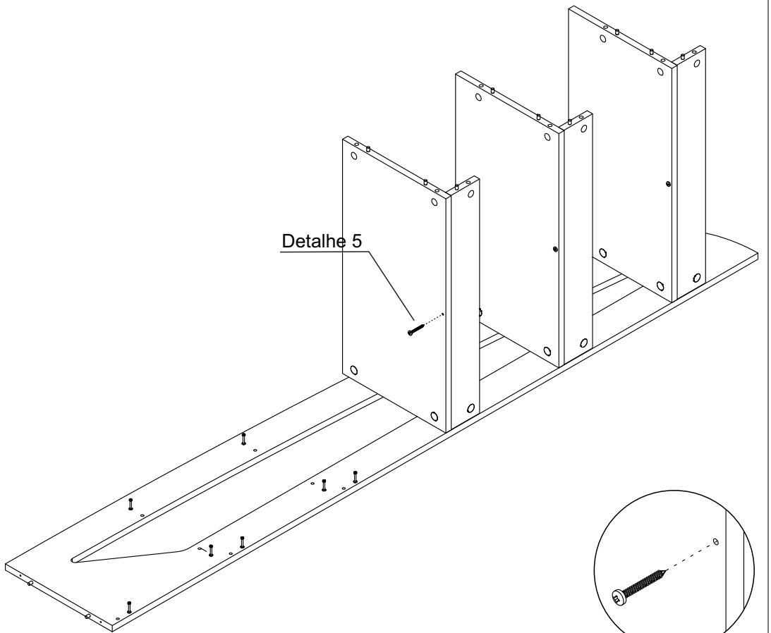
Detalhe 5 Detail/Detalle
