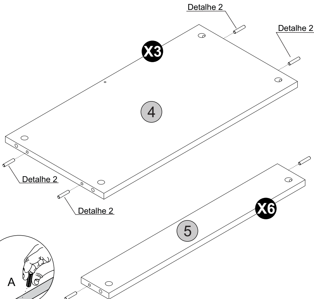
Detalhe 2 Detail/Detalle
