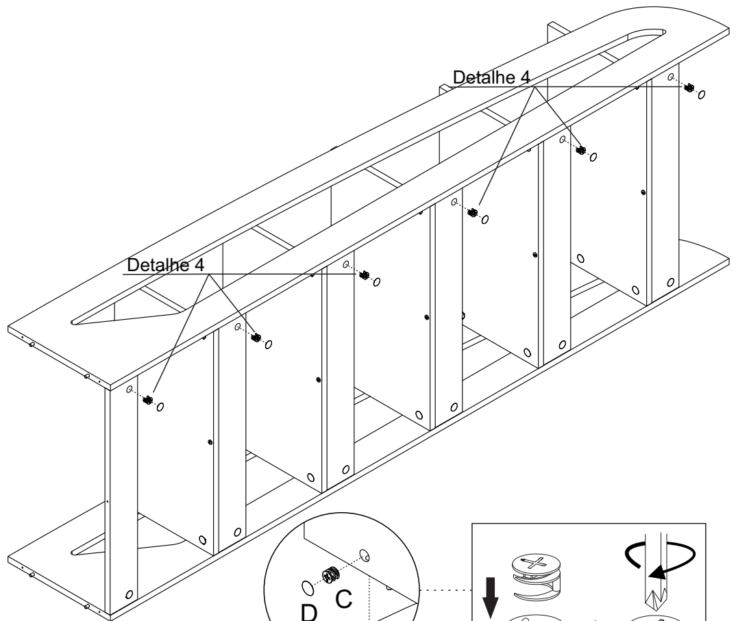
Detalhe 4 Detail/Detalle
