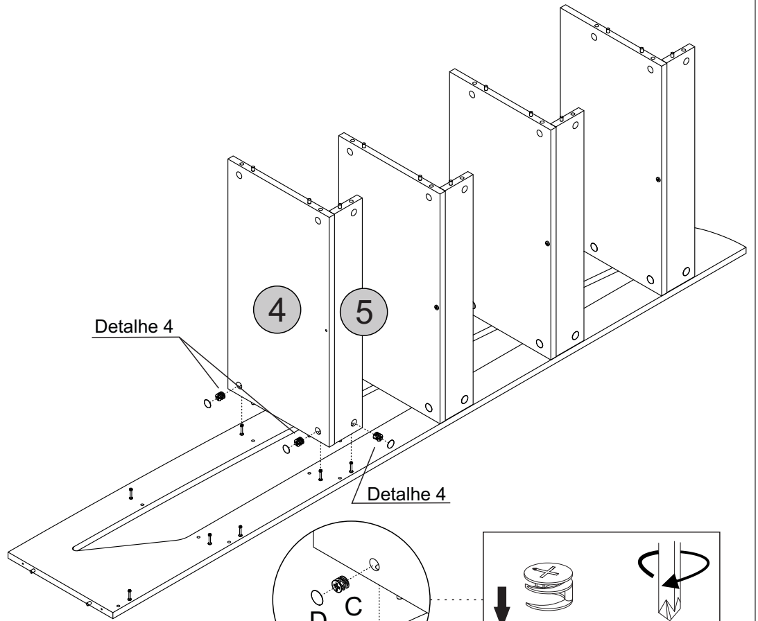
Detalhe 4 Detail/Detalle
