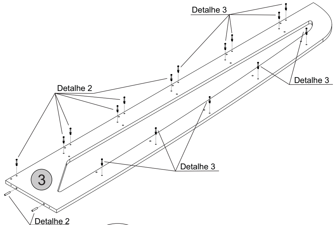
Detalhe 2 Detail/Detalle
