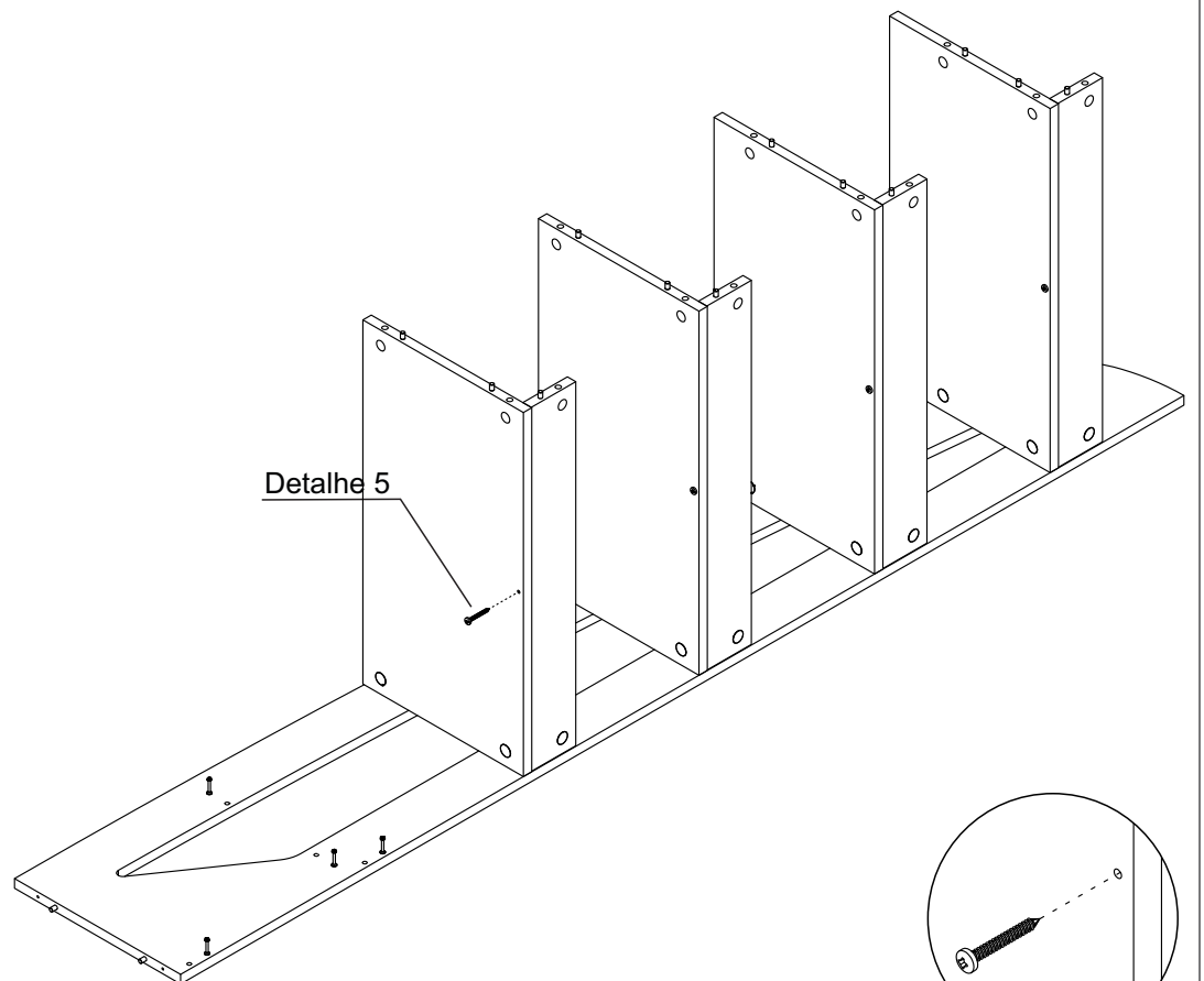
Detalhe 5 Detail/Detalle
