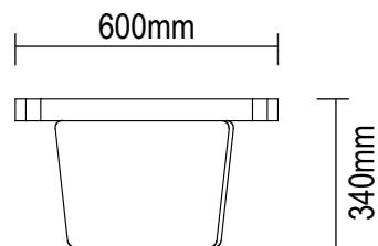
lateral/lado/side
