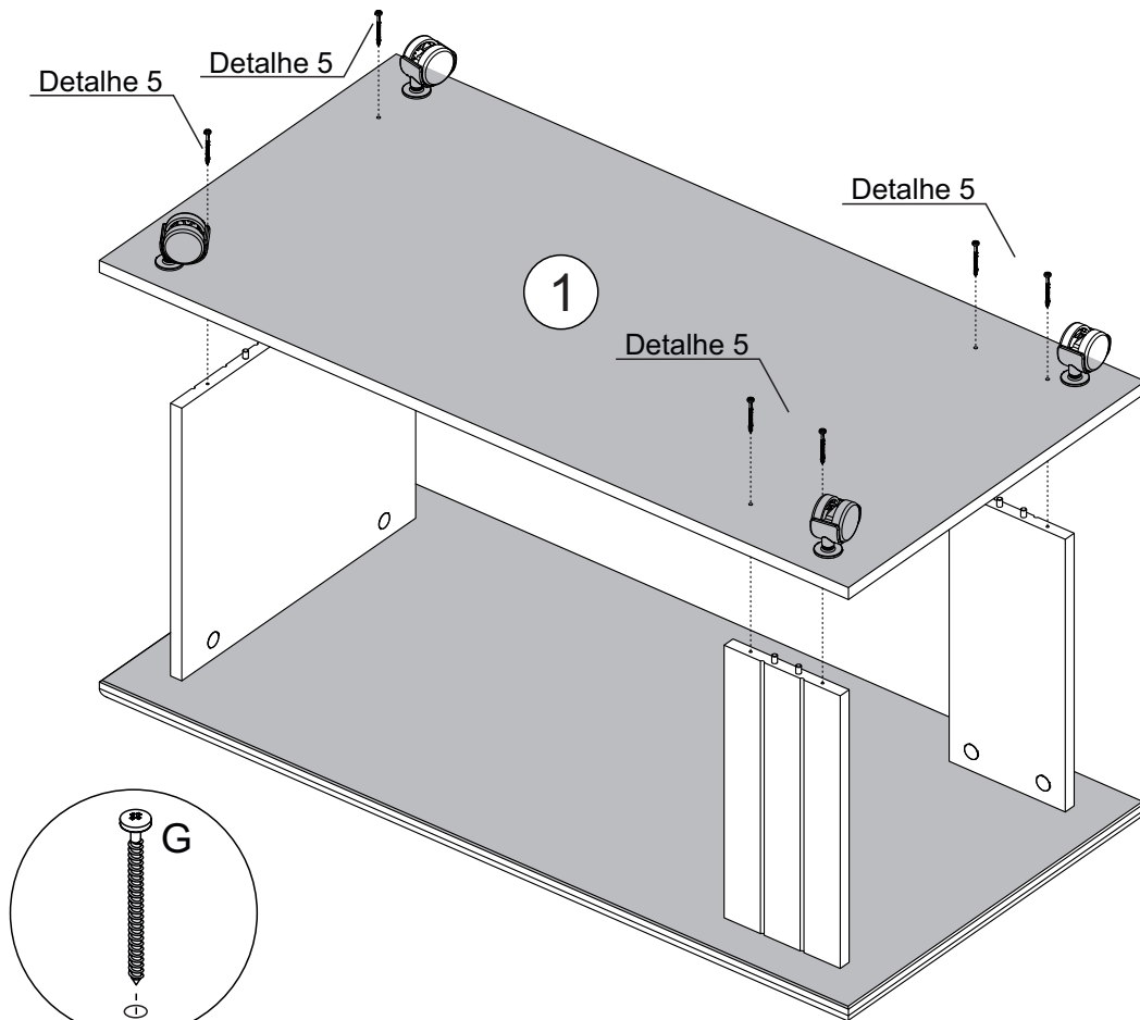
Detalhe 5 Detail/Detalle
