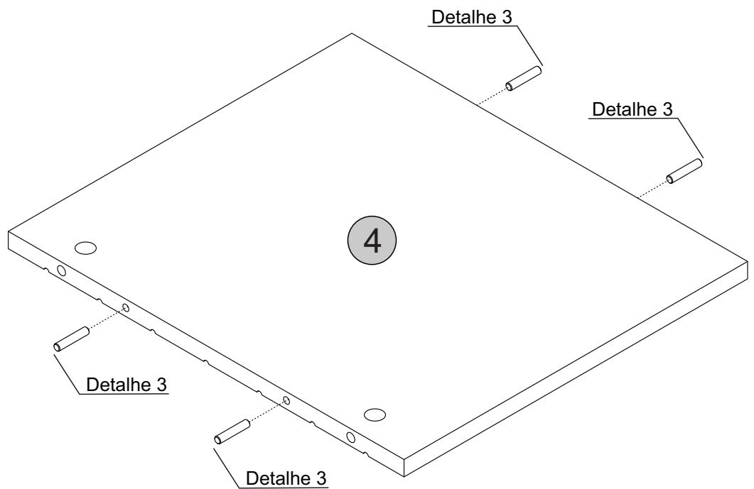
Detalhe 3 Detail/Detalle
