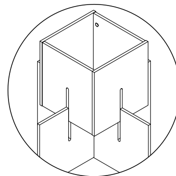
Detalhe 8 Detail/Detalle
