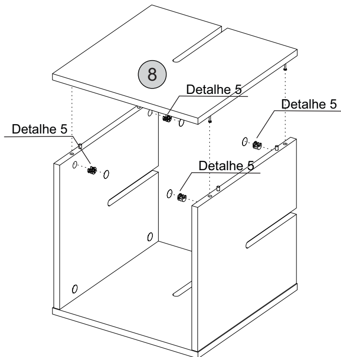
Detalhe 5 Detail/Detalle
