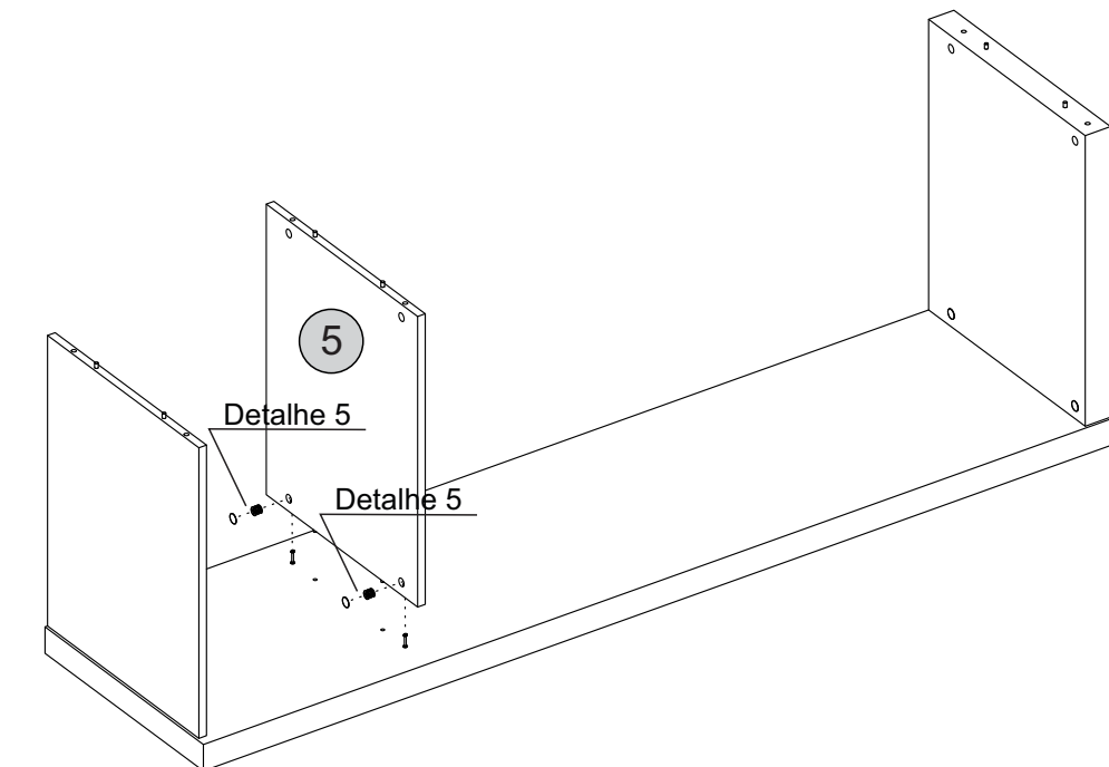
Detalhe 5 Detail/Detalle
